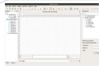
Interfață
